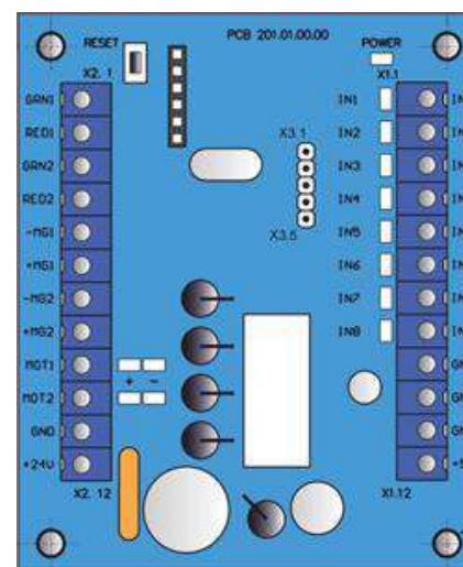
Рис. 9 – Зовнішній вигляд контролера моторизованого механізму РСВ.201.01.00.00
