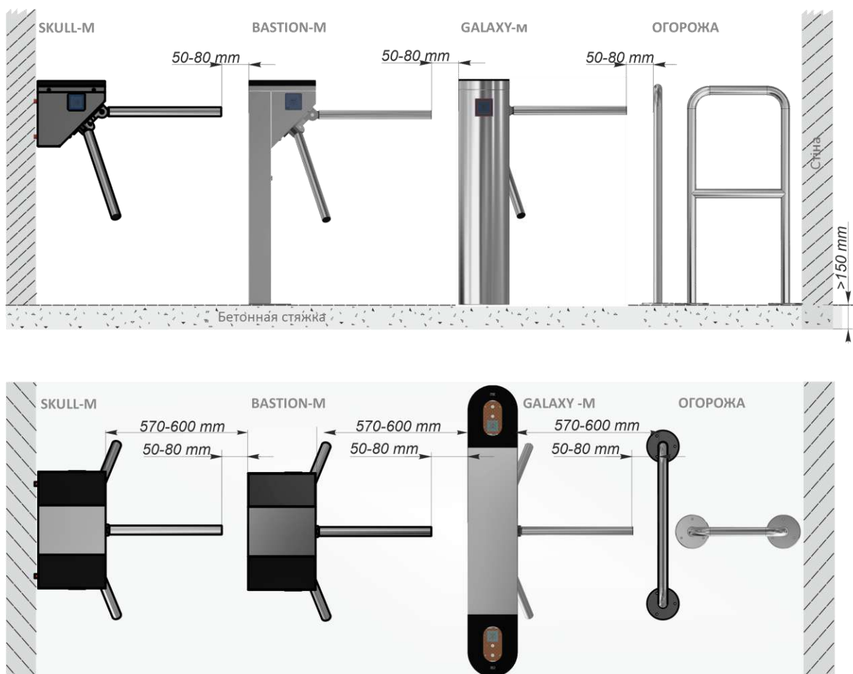
Рис.12 – Інсталяція розміщення турнікетів-триподів (умовно)
