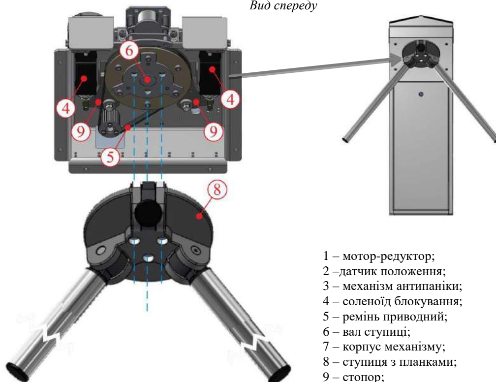
Рис. 5 – Робочий механізм турнікета
