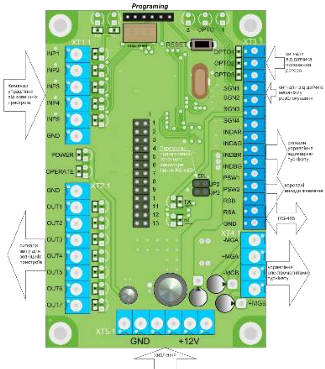
Рис. 8– Зовнішній вигляд контролера PCB.112.21.20.01
