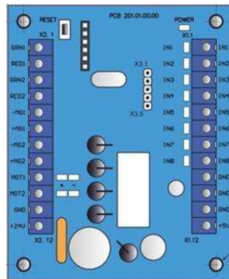
Рис. 9 – Зовнішній вигляд контролера РСВ.201.01.00.00 моторизованого механізму ротора (і хвртки)
