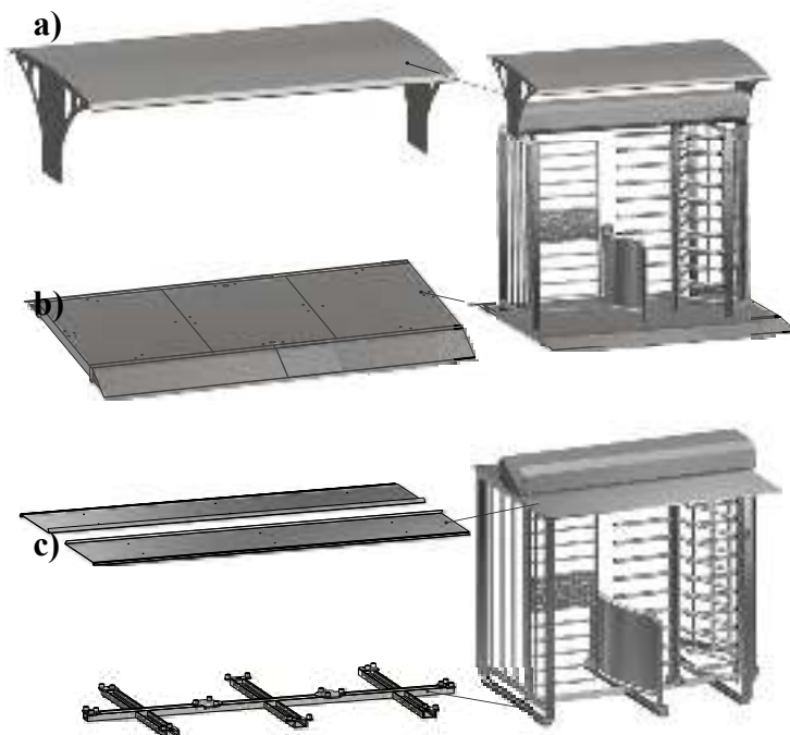
Рис.13– Використання додаткових елементів конструкції турнікету «BICYCLONE»
