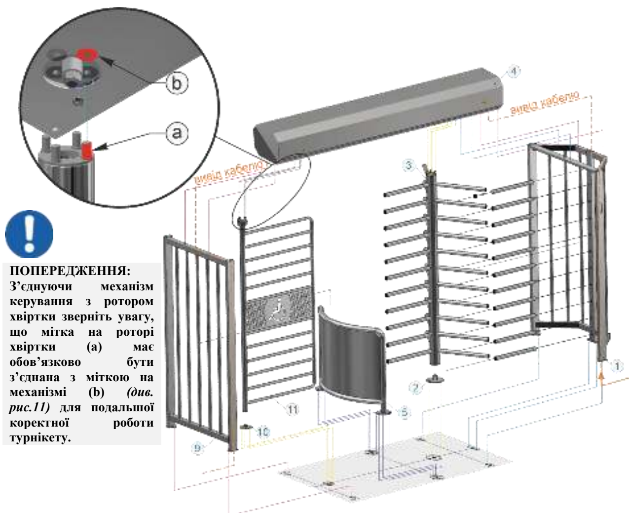
Рис. 11- Загальний вигляд встановлення турнікету «BICYCLONE» в проектне положення
