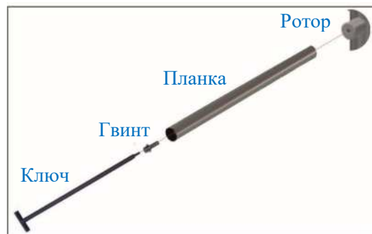
Рис.11– Складання основних елементів та встановлення планок турнікету
