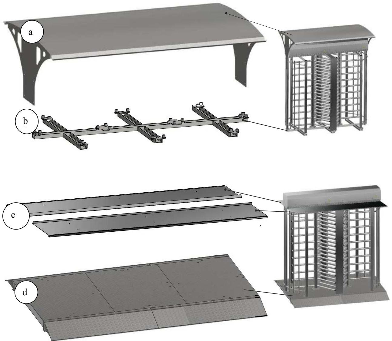
Рис.13– Використання додаткових елементів конструкції турнікета «SESAME-A TWIN»
