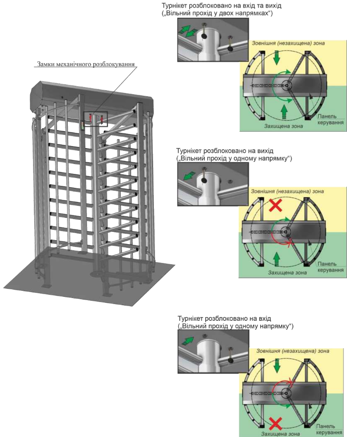
Рис.17– Принцип роботи механічного розблокування повнозростових турнікетів «SESAME-A»
