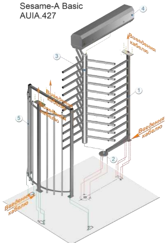
Рис. 9- Загальний вигляд встановлення турнікету «SESAME-A» і «SESAME-A BASIC» в проектне положення
