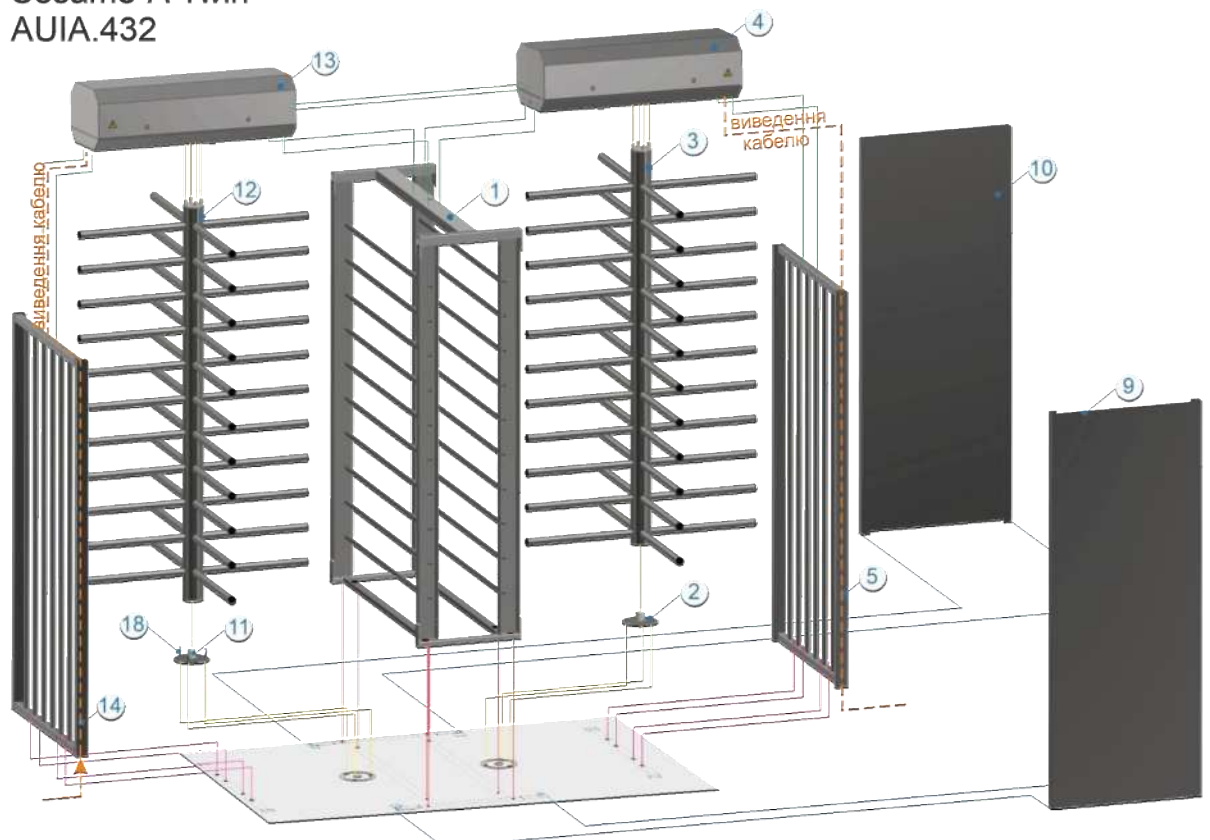
Рис. 10- Загальний вигляд встановлення турнікету «SESAME-A TWIN» в проектне положення
