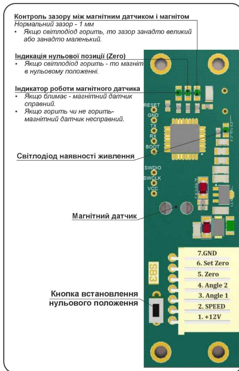
Рис. 19 – Опис контролера магнітного датчика
