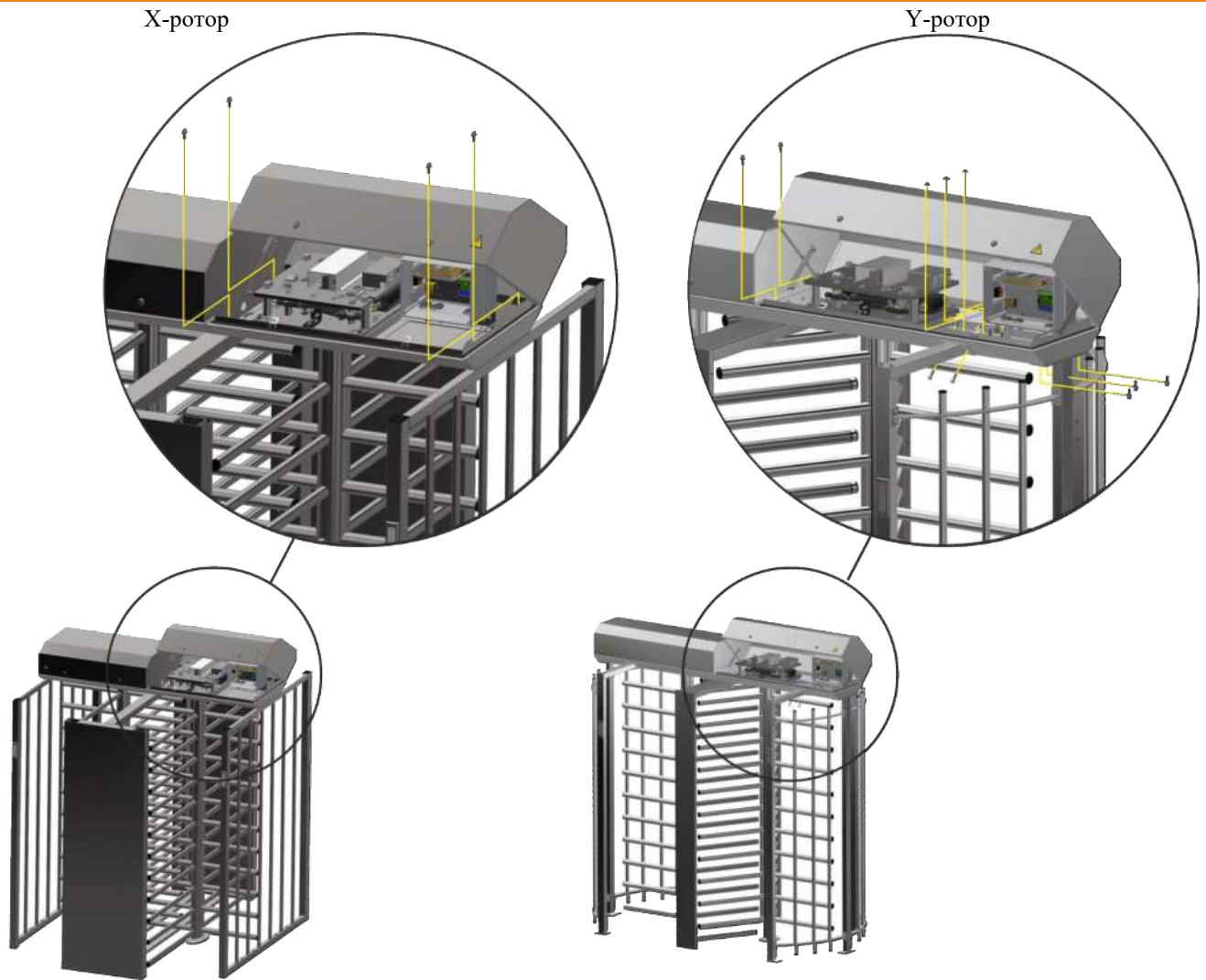
Рис.12- Кріплення контейнера
