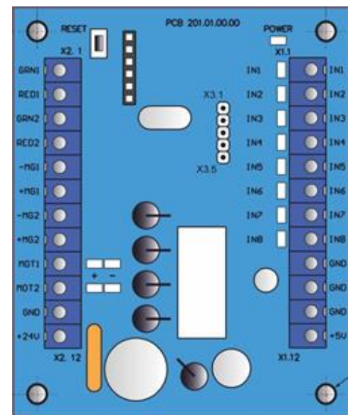
Рис. 7 - Зовнішній вигляд контролера моторизованого механізму PCB.201.01.00.00
