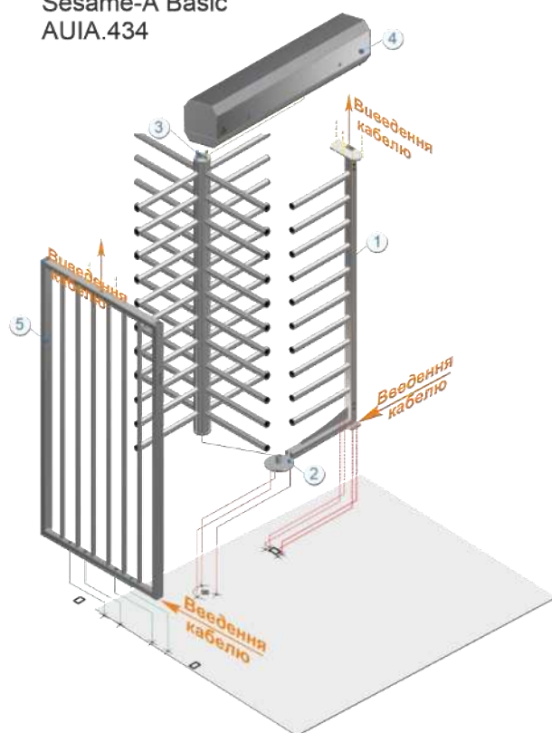
Рис. 9- Загальний вигляд встановлення турнікету «SESAME-A» і «SESAME-A BASIC» в проектне положення
