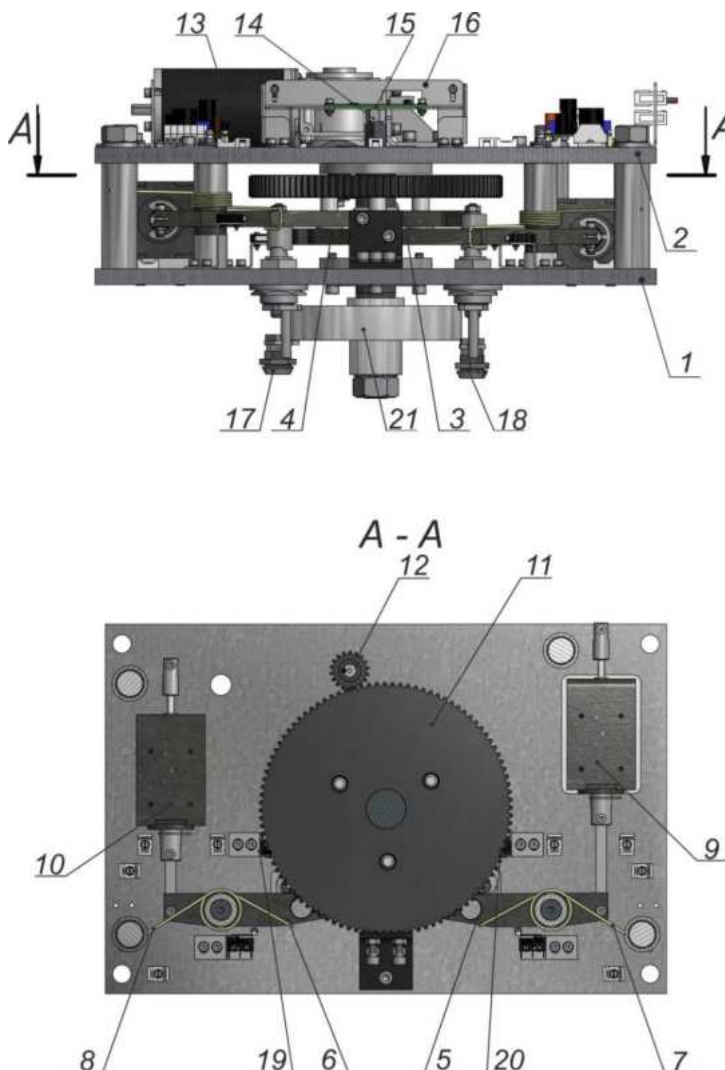
Рис. 4 – Конструкція механізму керування ротором
