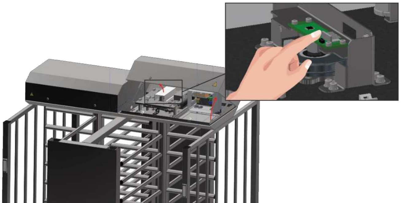
Рис.18 - Налаштування нульового положення
