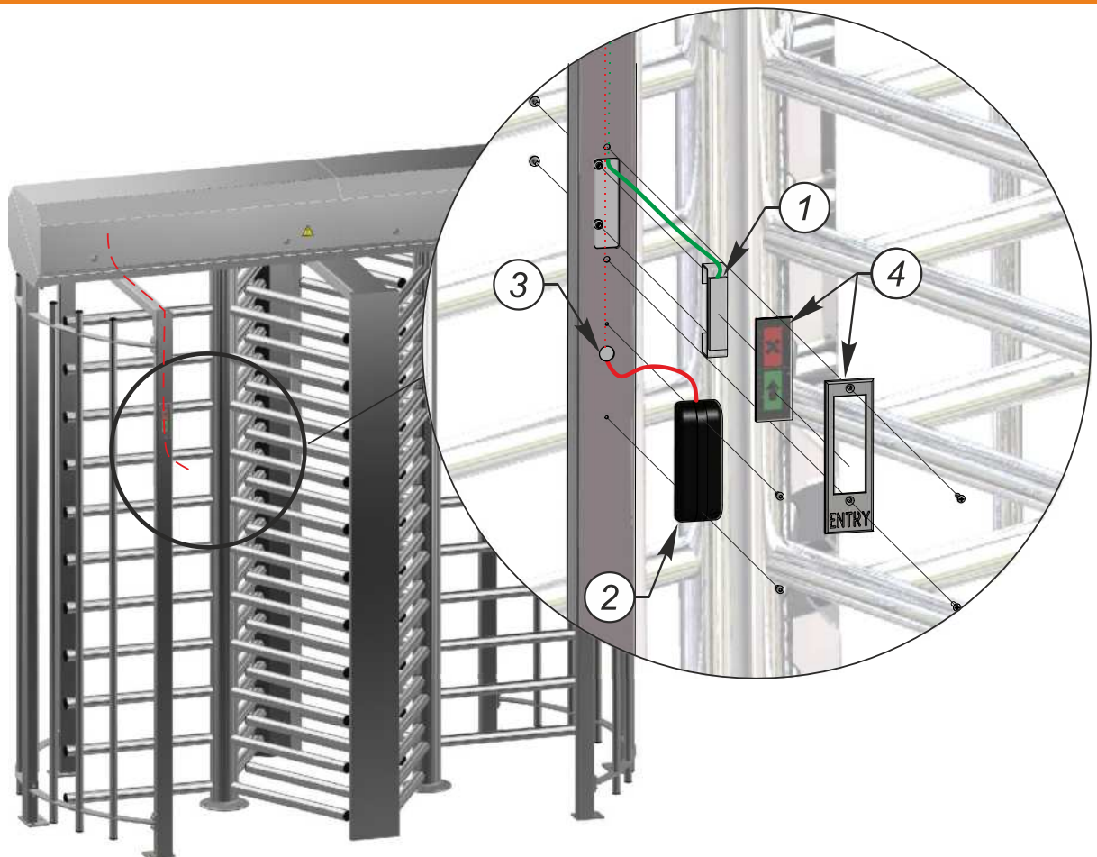
Рис.14 - Встановлення зчитувача безконтактних карт та табло індикації
